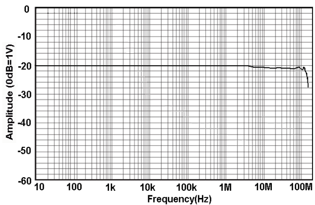
图 1.b HCP8030D 幅频曲线
