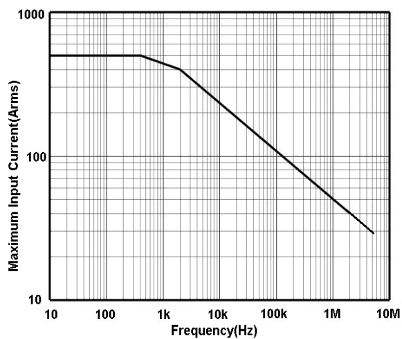
图 14 HCP8500 最大测量电流 VS 频率曲线 (超过该曲线所示最大电流连续使用会导致探头烧毁)
