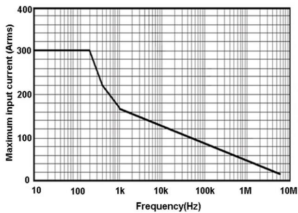
图 11 HCP8300 最大测量电流 VS 频率曲线 (超过该曲线所示最大电流连续使用会导致探头烧毁)
