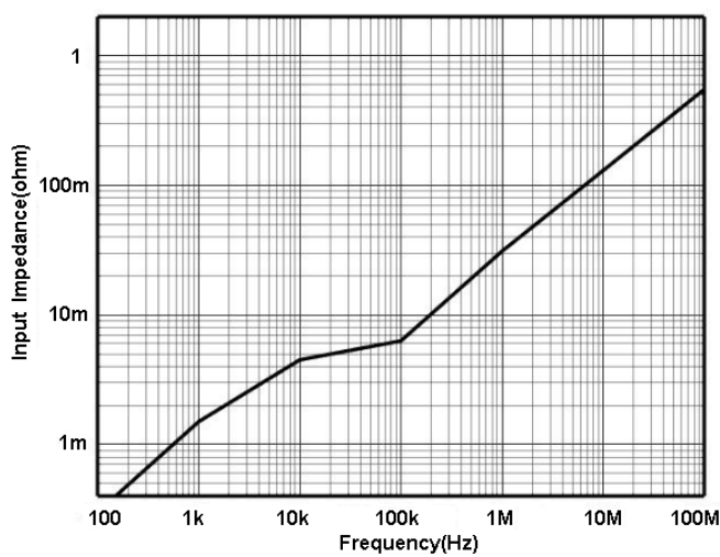
图 3.b HCP8030D 输入阻抗 VS 频率曲线
