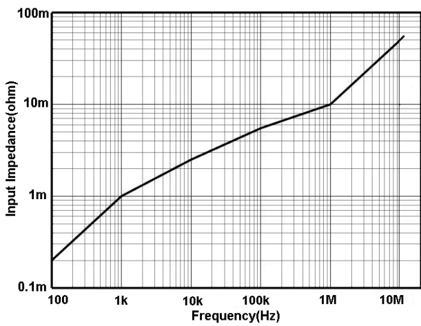
图 9 HCP8150 输入阻抗 VS 频率曲线
