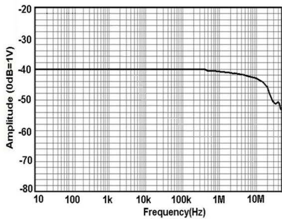
图 10 HCP8300 幅频曲线
