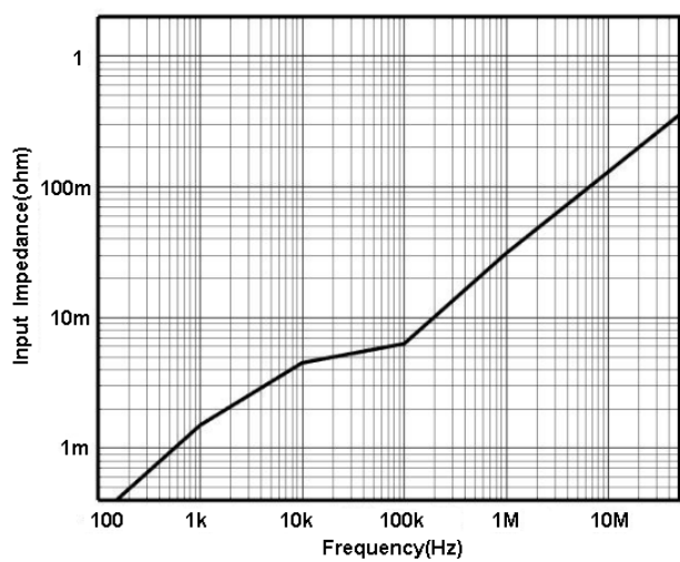
图 3.a HCP8030 输入阻抗 VS 频率曲线
