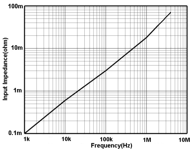
图 15 HCP8500 输入阻抗 VS 频率曲线
