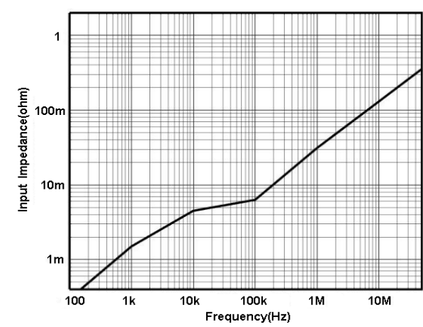
图 6 HCP8050 输入阻抗 VS 频率曲线
