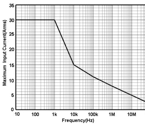
图 2.a HCP8030 最大测量电流 VS 频率曲线 (超过该曲线所示最大电流连续使用会导致探头烧毁)
