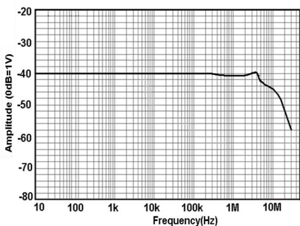
图 13 HCP8500 幅频曲线
