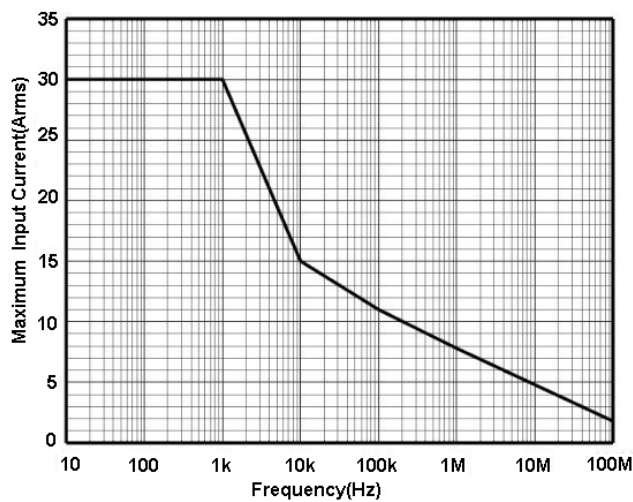
图 2.b HCP8030D 最大测量电流 VS 频率曲线 (超过该曲线所示最大电流连续使用会导致探头烧毁)
