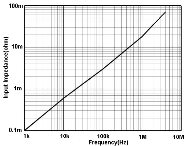
图 12 HCP8300 输入阻抗 VS 频率曲线
