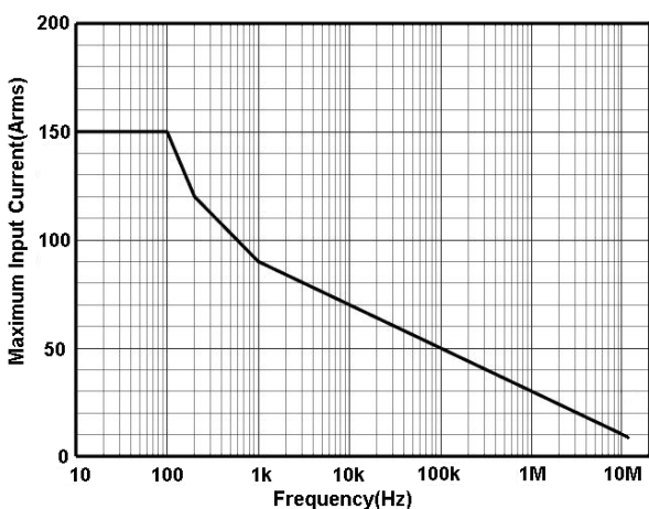
图 8 HCP8150 最大测量电流 VS 频率曲线 (超过该曲线所示最大电流连续使用会导致探头烧毁)
