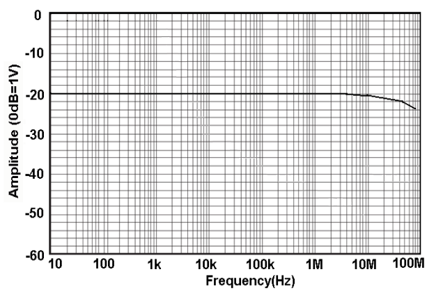
图 4 HCP8050 幅频曲线
