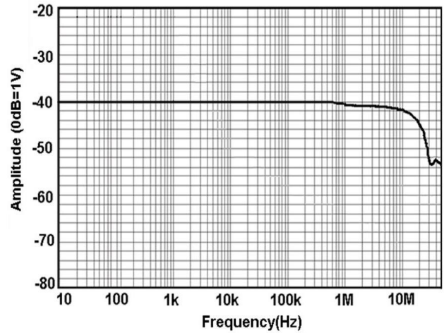
图 7 HCP8150 幅频曲线
