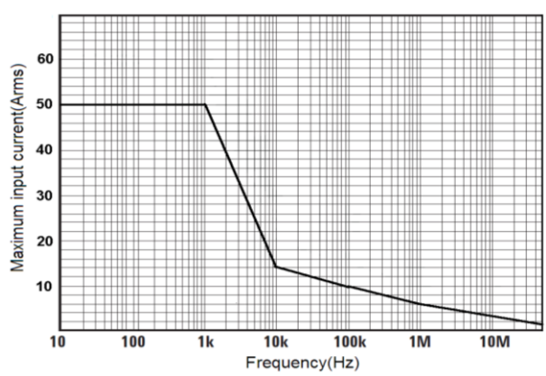
图 5 HCP8050 最大测量电流 VS 频率曲线 (超过该曲线所示最大电流连续使用会导致探头烧毁)
